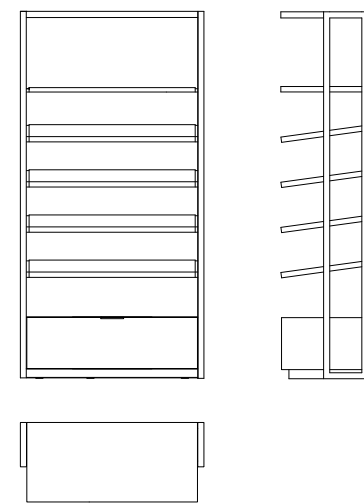
MODULE D 120 Modulo D 120
