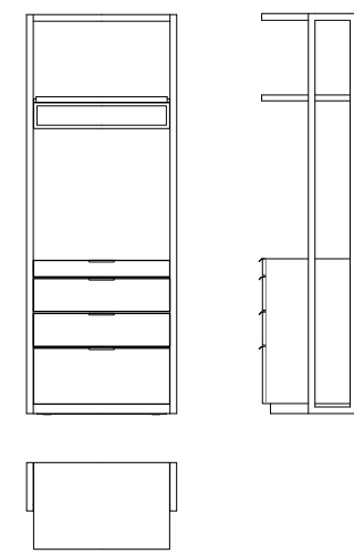
MODULE B 90 Modulo B 90
